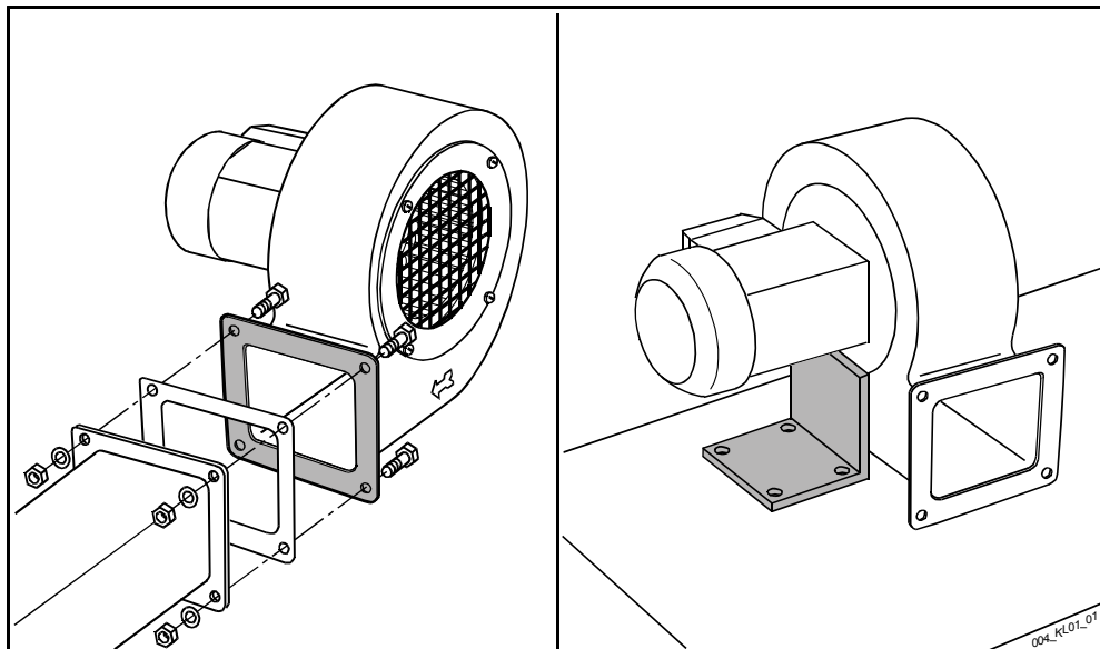
Am Ausblasflansch
