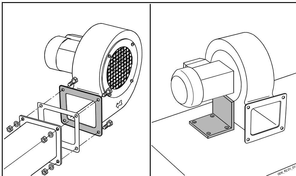
Vid utblåsningsflänsen
