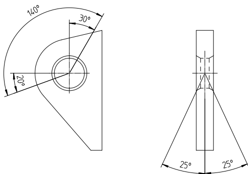
zulässige Belastungsrichtungen
